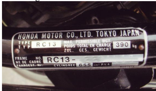
Eventuale targhetta identificativa
